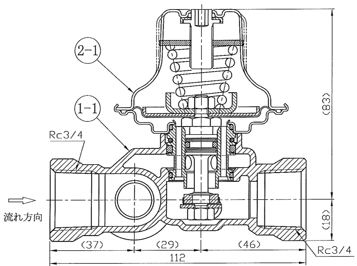
AA断面図(S=1:1)
